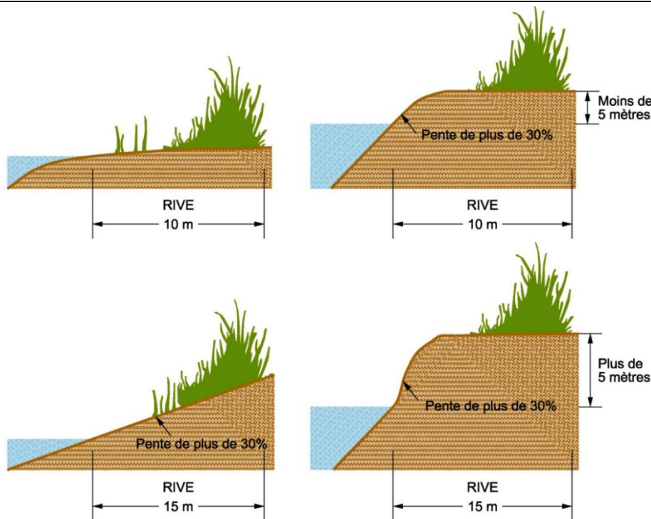
Croquis 17.1 Détermination de la largeur de la rive selon la pente de la rive
