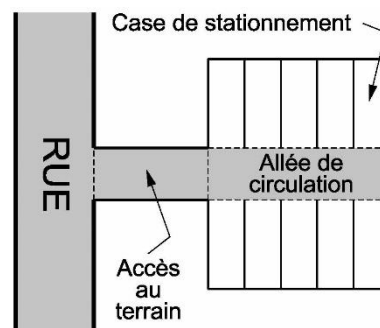
Croquis 2.1 : Parties d'une aire de stationnement
